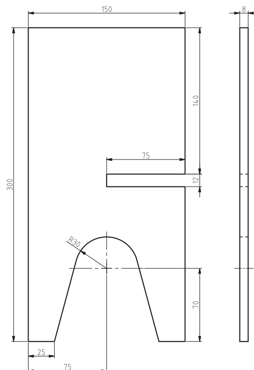
شکل ۶-۹. نقشهٔ یکی از قطعه‌های رحل قرآن
